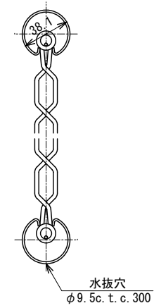
洞縁に金網取付断面図 S=1:3
