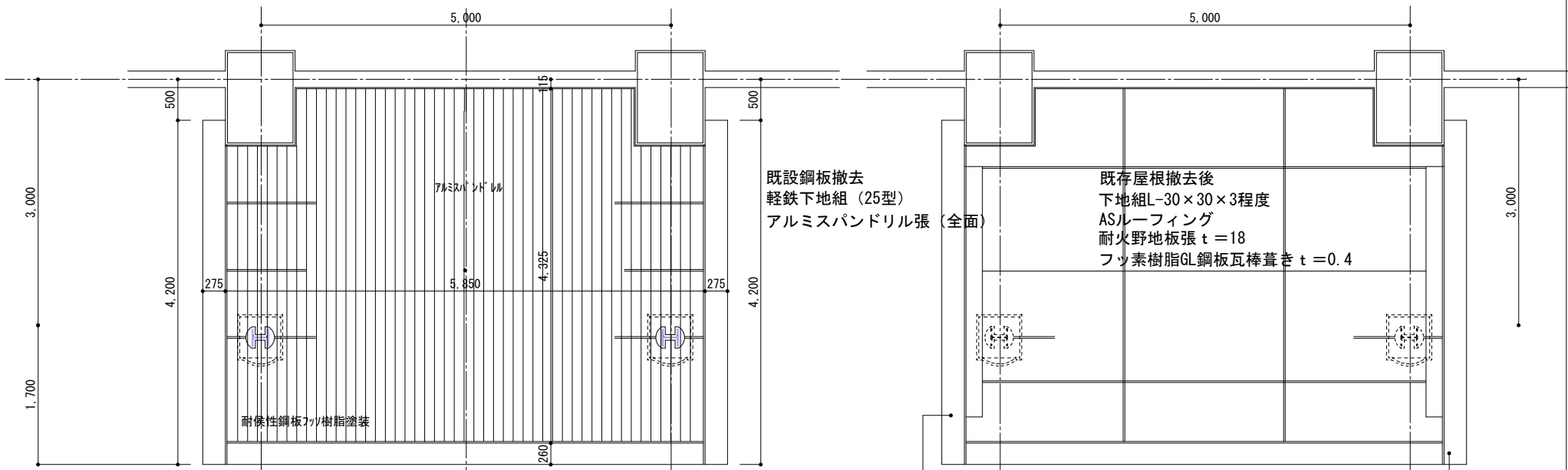
玄関廻り2階天井伏図 1/50
