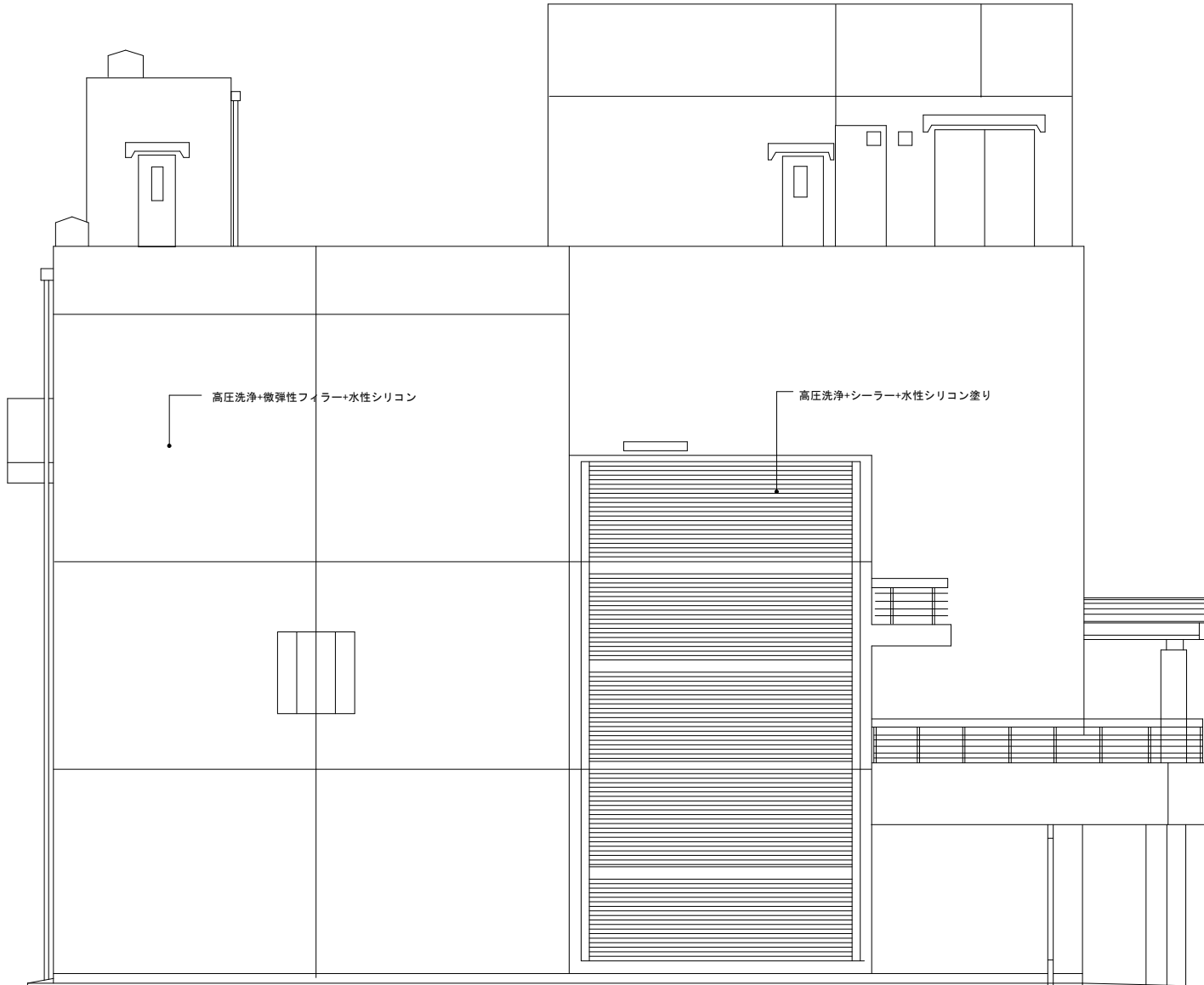
西立面図 1/100
