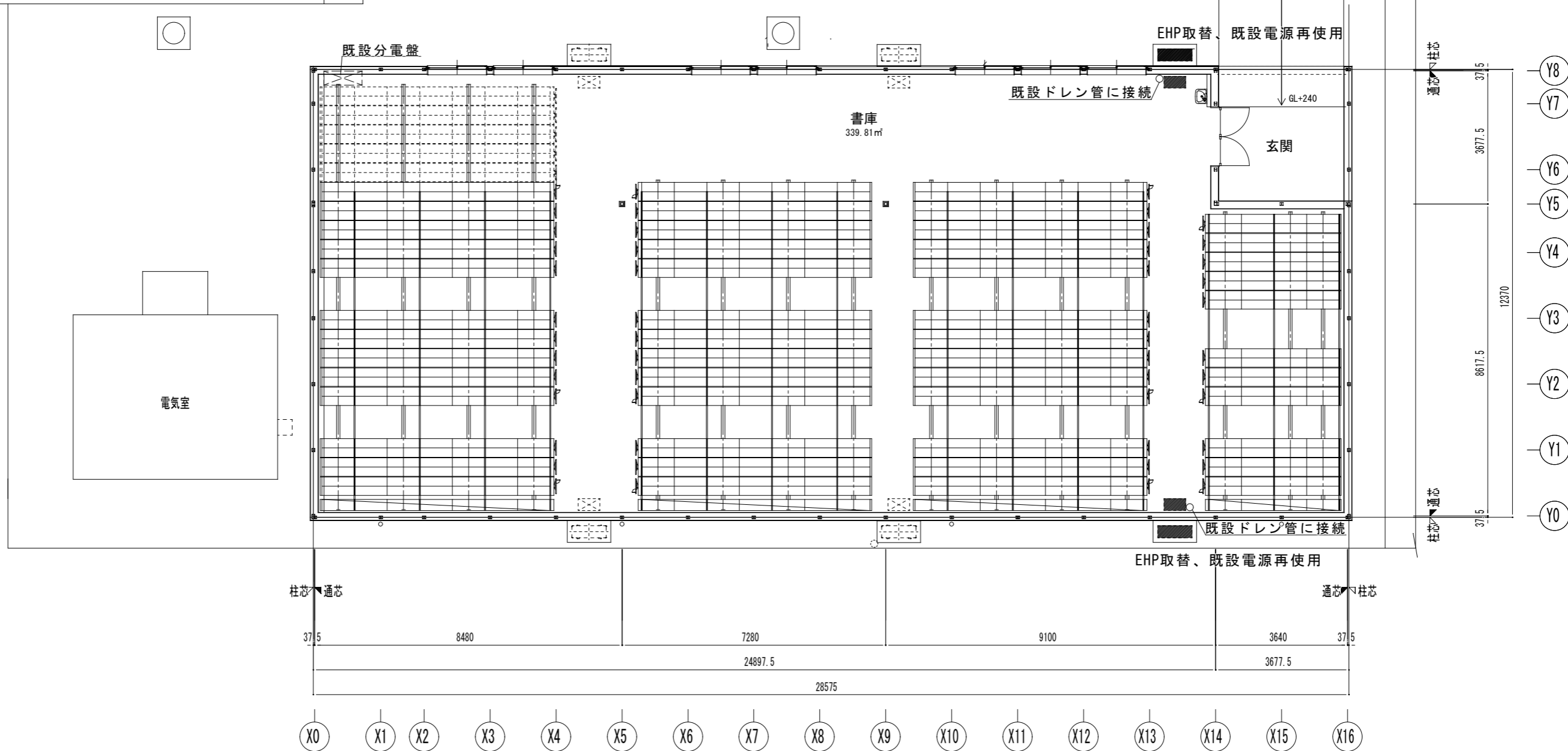
平面図
